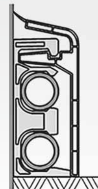
Schnittzeichnung der mit Leiste abgedeckten Rohre
